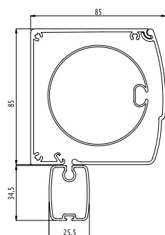
Fixscreen® 85
